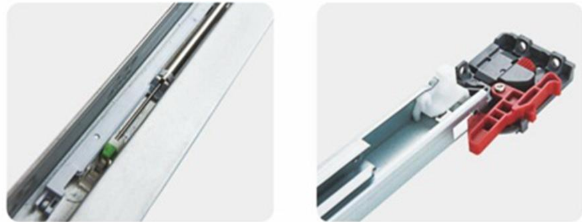
金属阻尼管 Metal damping tube 三维可调连接件 3D adjustment connector
